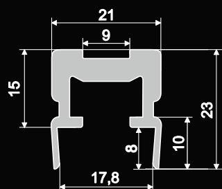
Paraván csatlakozó profil 20x20 mm -es oszlophoz
