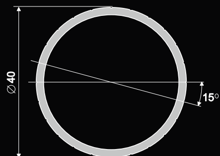
Paraván oszlop Ø40 mm
